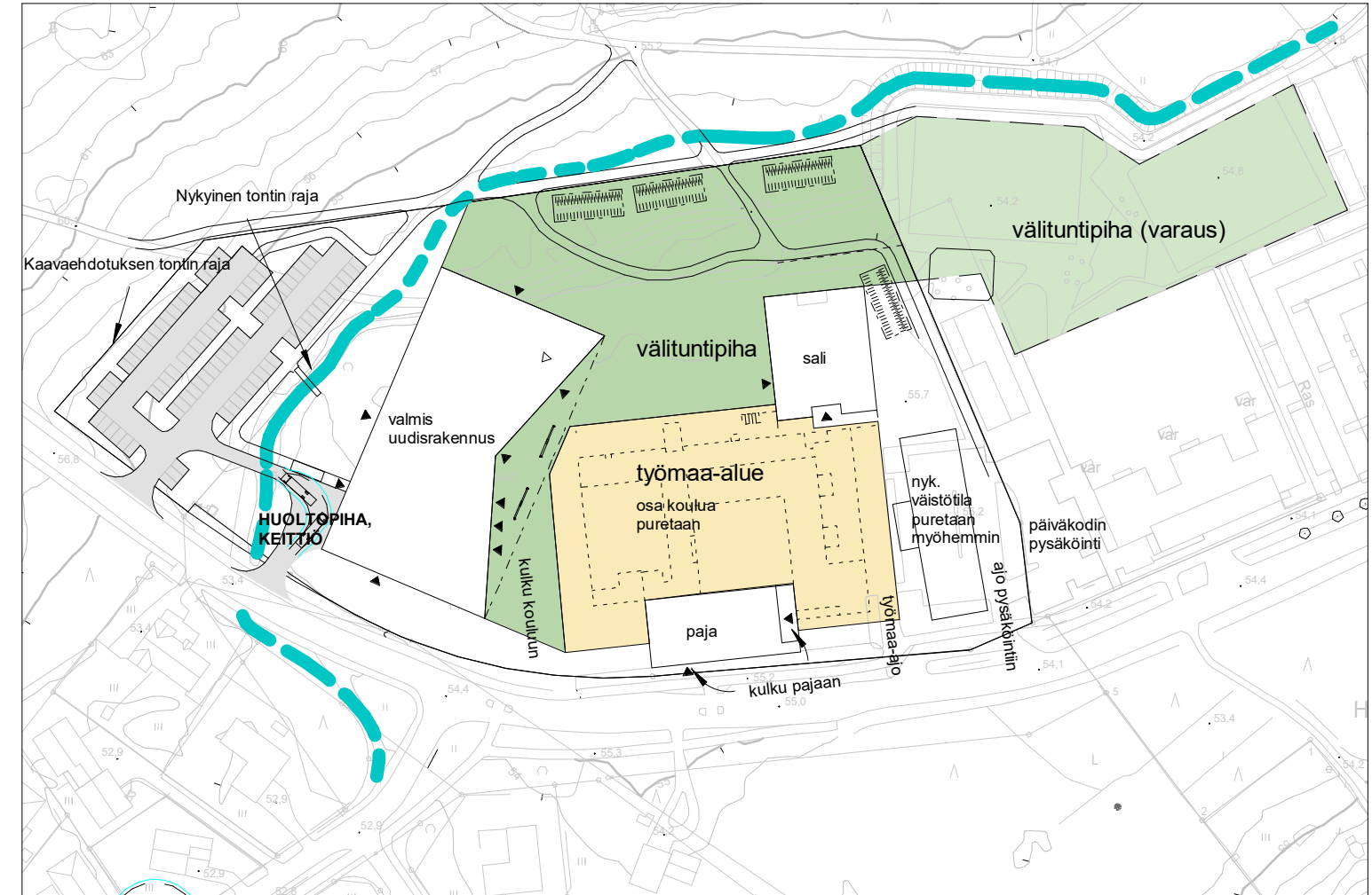
LUONNOS asemapiirros PURKU 1 : 2000
