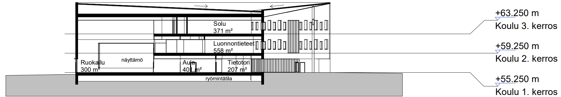
Leikkaus A 1 : 450
